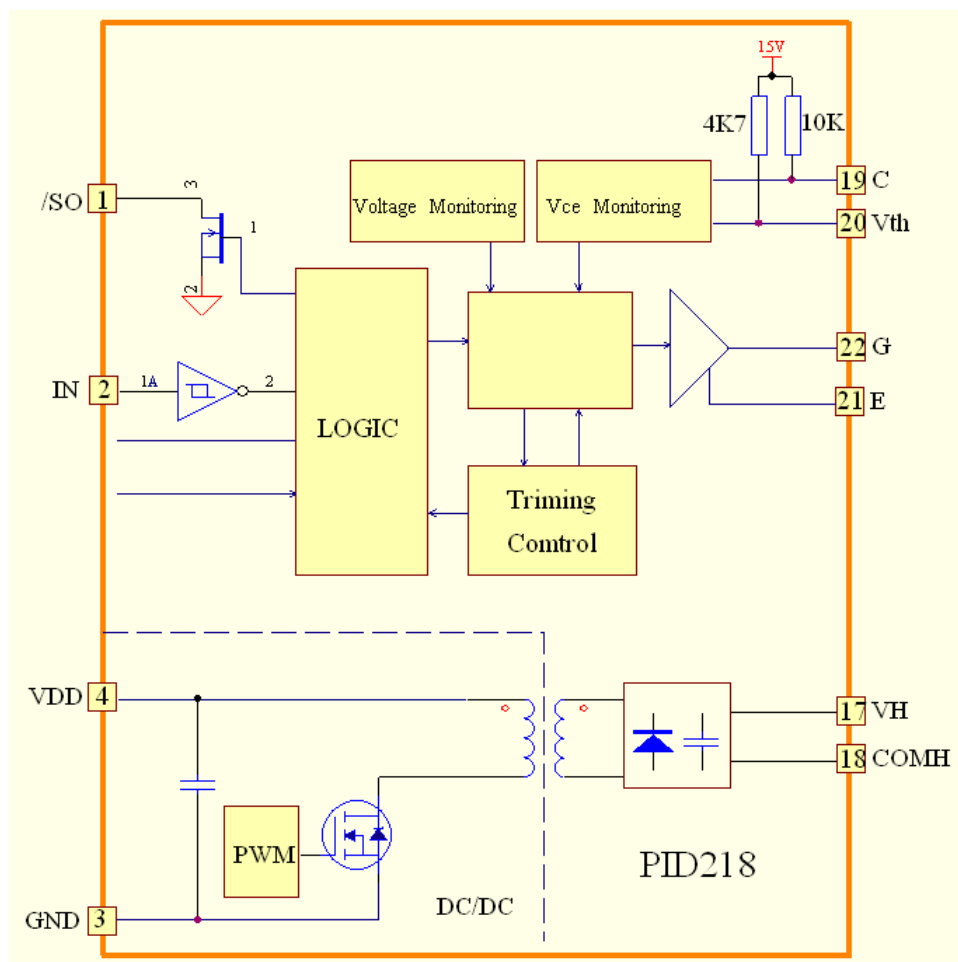
PID218 结构原理图
