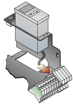
比调仪安装示例
