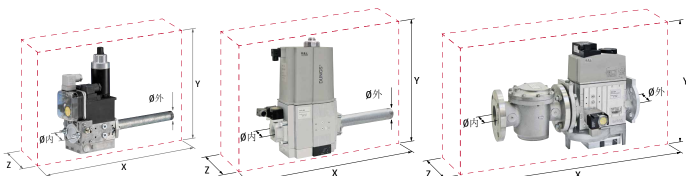
MB型“一体式”燃气阀组示例
