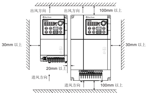
图 2-3 两台变频器左右安装
