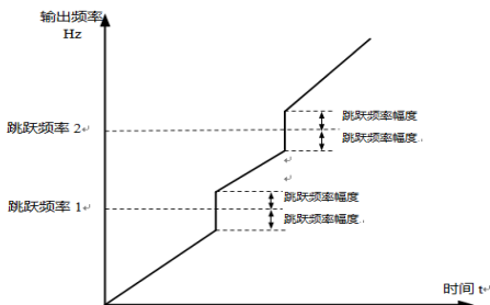
图 6-8-3 加减速过程中跳跃频率有效示意图
