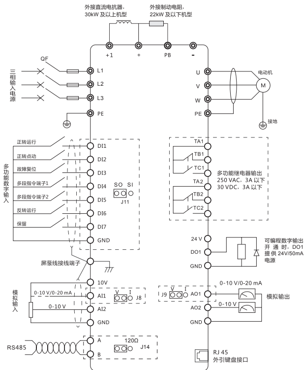
图 2-9 G1 系列变频器系统配线图
