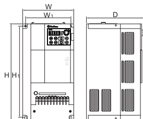
图 C-6 框架 D 安装尺寸
