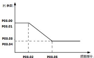
图 6-3-1 PI 参数示意图
