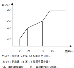
图 6-4-2 多点 V/F 曲线设定示意图
