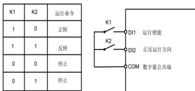
图 6-5-2 两线式模式 2
