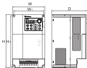
图 C-4 框架 B 安装尺寸
