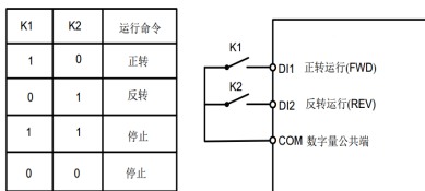
图 6-5-1 两线式模式 1
