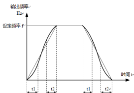
图 6-1-1 S 曲线加减速 A 示意图
