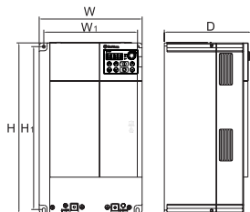
图 C-8 框架 F 安装尺寸
