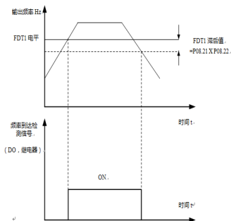
图 6-8-5 FDT1 电平示意图
