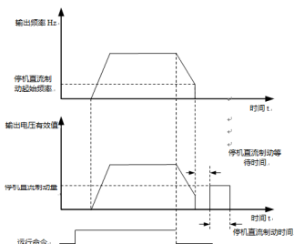
图 6-1-3 停机直流制动示意图
