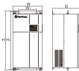
图 C-10 框架 H 安装尺寸
