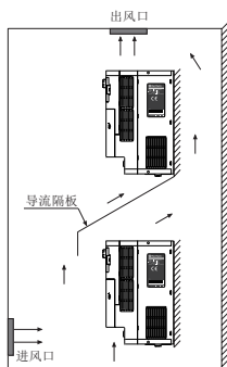
图 2-2 两台变频器上下安装
