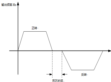
图 6-8-4 正反转死区时间示意图
