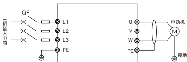
图 4-1 试运行接线图
