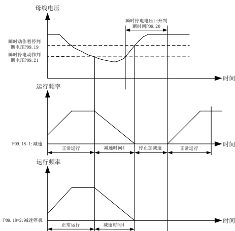
图 6-9-3 瞬时停电动作示意图
