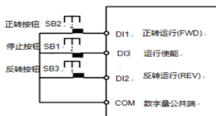
图 6-5-3 三线式控制模式 1
