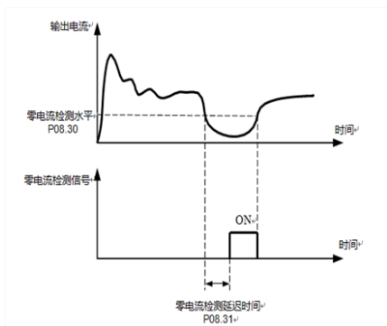
图 6-8-8 零电流检测示意图
