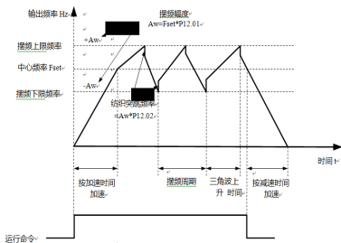
图 6-12-1 摆频工作示意图
