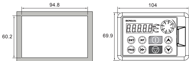
图 C-2 键盘底座安装尺寸 (单位: mm)
