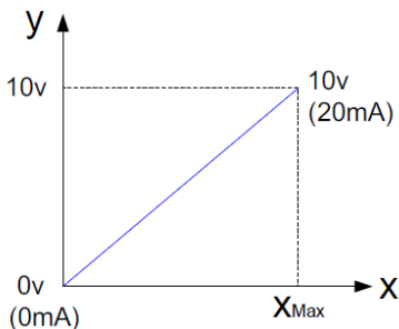
图 6-6-1 无零偏或增益时的输出示意图
