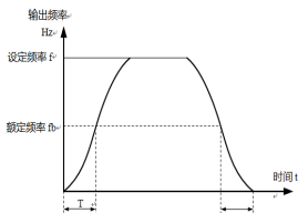
图 6-1-2 S 曲线加减速 B 示意图
