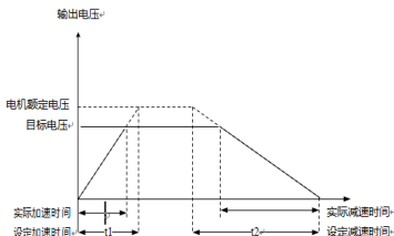
图 6-4-3 V/F 分离示意图
