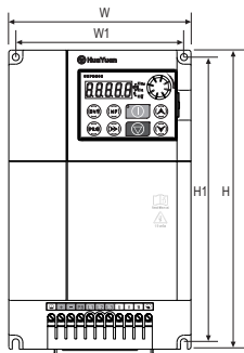
图 2-4 壁挂式安装示意图
