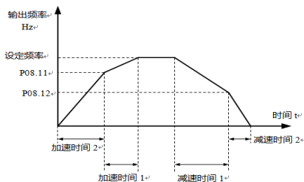
图 6-8-1 加减速时间切换示意图
