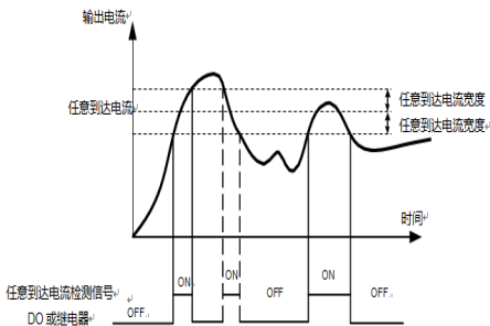
图 6-8-10 任意到达频率检测示意图
