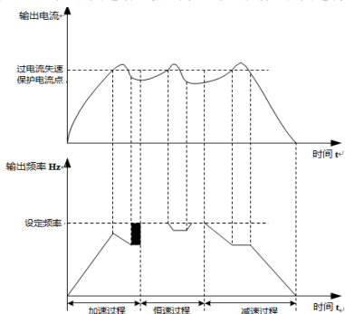
图 6-9-2 过流失速保护示意图
