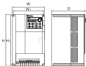
图 C-5 框架 C 安装尺寸
