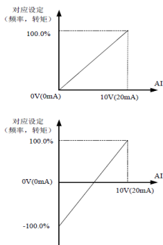
图 6-5-6 模拟给定与设定量的对应关系
