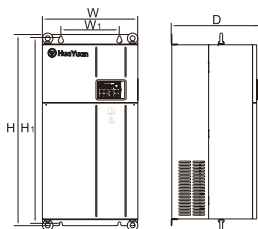
图 C-11 框架 J 安装尺寸
