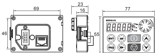
图 C-1 键盘安装尺寸 (单位: mm)
