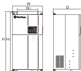
图 C-9 框架 G 安装尺寸
