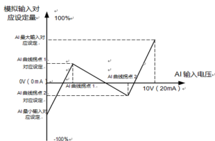
图 6-5-7 曲线 4 和曲线 5 的示意图
