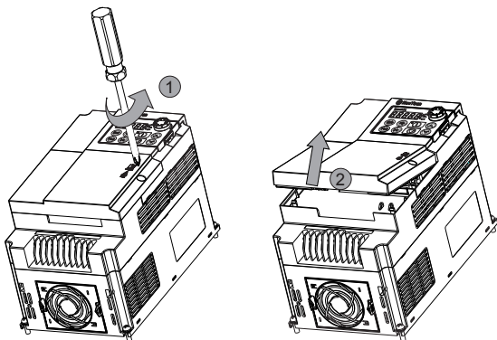
图 2-7 端子盖的拆卸
