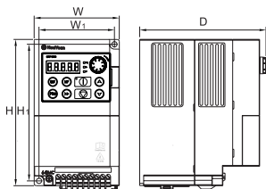
图 C-3 框架 A 安装尺寸
