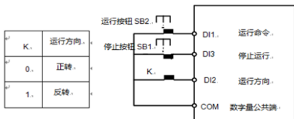
图 6-5-4 三线式控制模式 2
