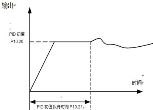
图 6-10-3 PID 初值功能示意图
