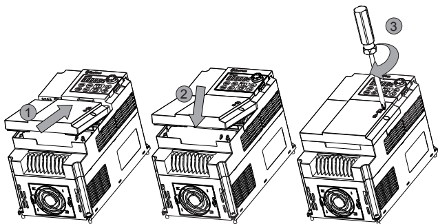
图 2-8 端子盖的安装
