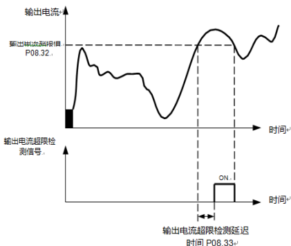
图 6-8-9 输出电流超限检测示意图
