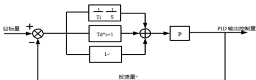
图 6-10-1 过程 PID 的控制原理框图
