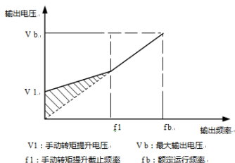
图 6-4-1 手动转矩提升示意图
