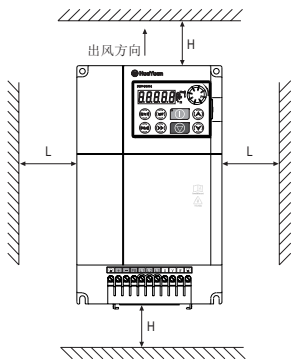
图 2-1 安装的间隔距离
