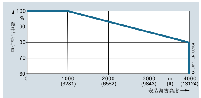
允许的输出现流, 随电源电压变化针对外形尺寸从 FSA 到 FSF 的功率模块 PM230
