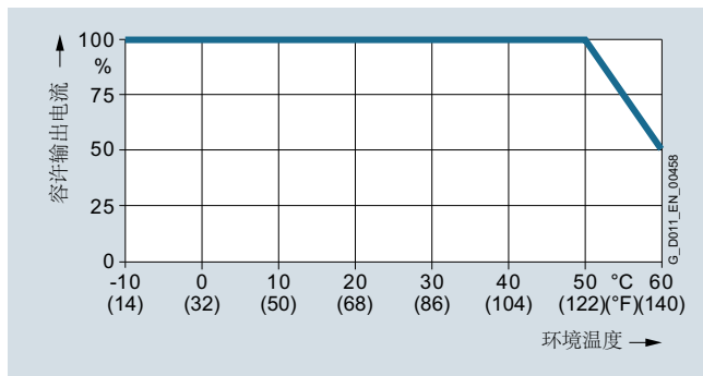
高过载 (HO) 时, 机座号为 FSA 至 FSC 的 PM230 电源模块的容许输出电流随环境温度的变化而变化
