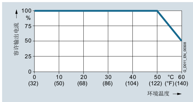
高过载 (HO) 时, 机座号为 FSD 至 FSF 的 PM230 电源模块的容许输出电流随环境温度的变化而变化
