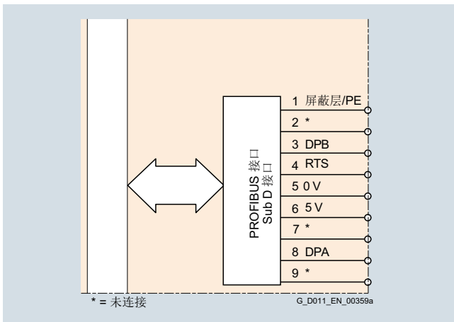
通讯接口 PROFIBUS DP
