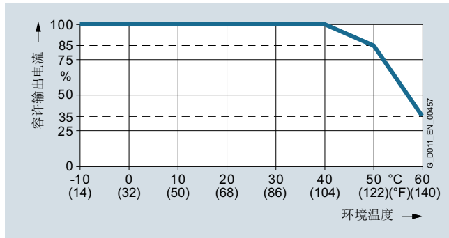
低过载 (LO) 时, 机座号为 FSA 至 FSC 的 PM230 电源模块的容许输出电流随环境温度的变化而变化
