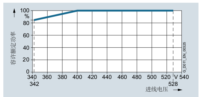
允许的额定功率, 随电源电压变化, 针对外形尺寸从 FSA 到 FSF 的功率模块 PM230
