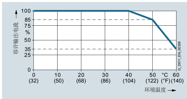
低过载 (LO) 时, 机座号为 FSD 至 FSF 的 PM230 电源模块的容许输出电流随环境温度的变化而变化
