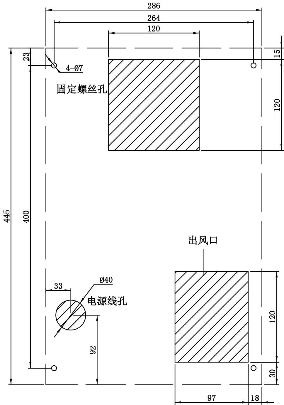
阴影部分开孔 柜外向内看
