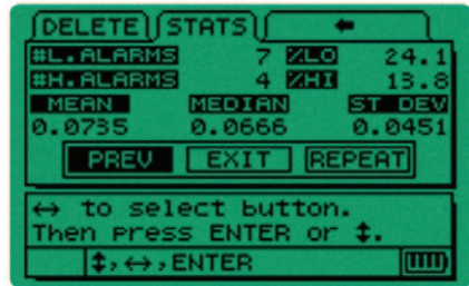
统计报告显示高/低报警、平均值、中位数和标准偏差。
