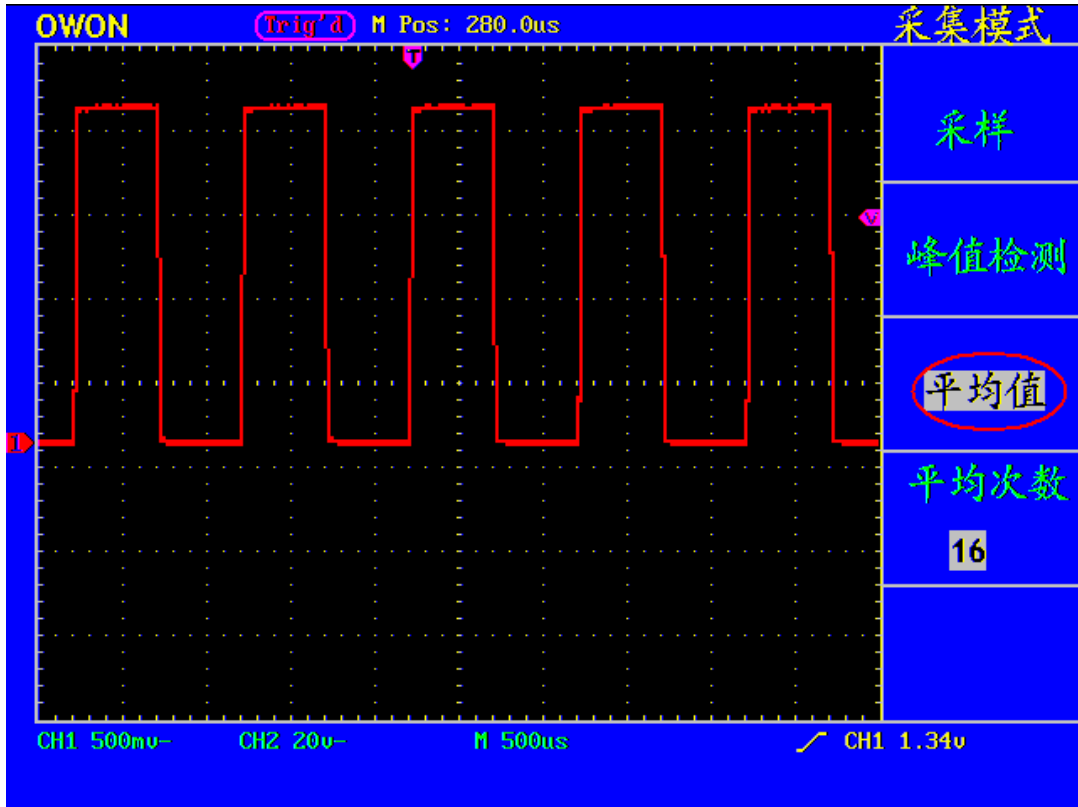
图 60： 去除噪声信号的波形
