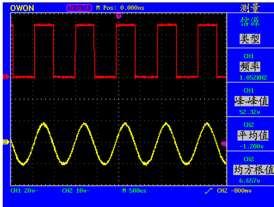
图50：自动测量
