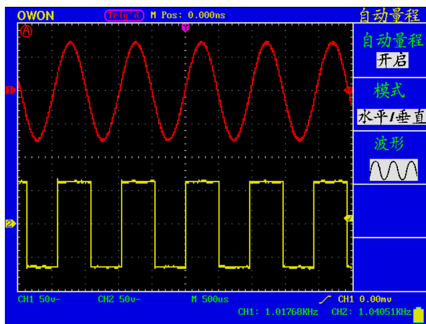
图 54 自动量程 水平/垂直模式多周期波形图
