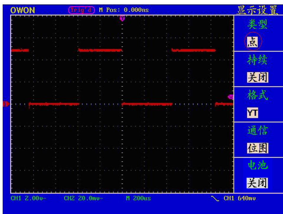
图 41： 点显示类型
