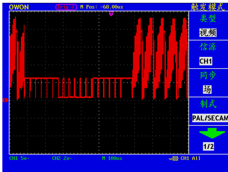
图 62 视频场触发波形
