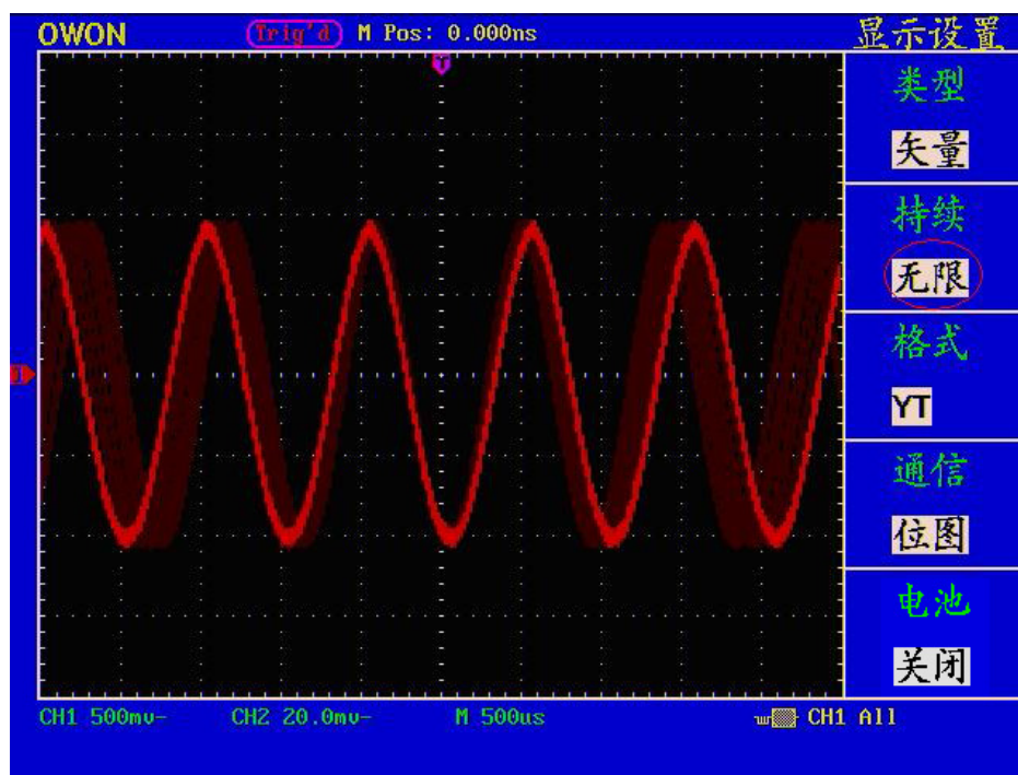
图42：无限余辉显示
