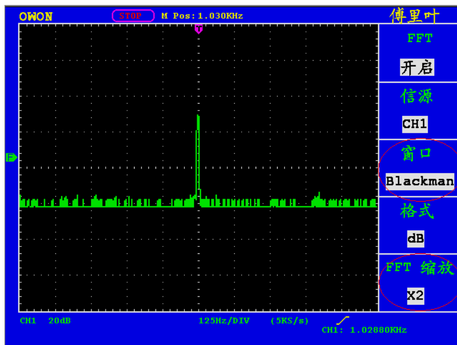
图21. Blackman窗
