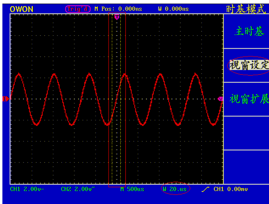
图 28: 视窗设定
