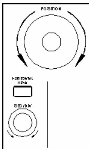
图12：水平控制区
