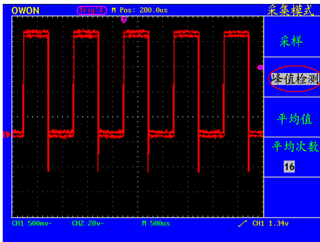
图 59： 含噪声信号的波形
