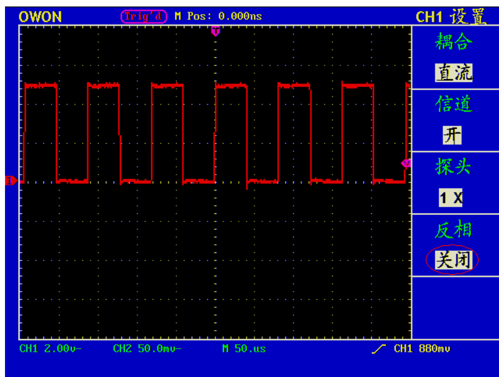
图 18 未反相的波形
