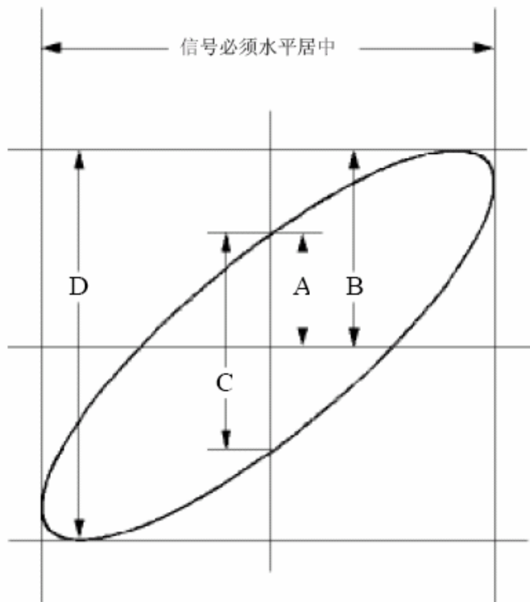
图 61 李沙育 (Lissajous) 图形
