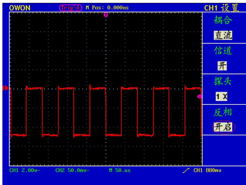
图 19 反相的波形
