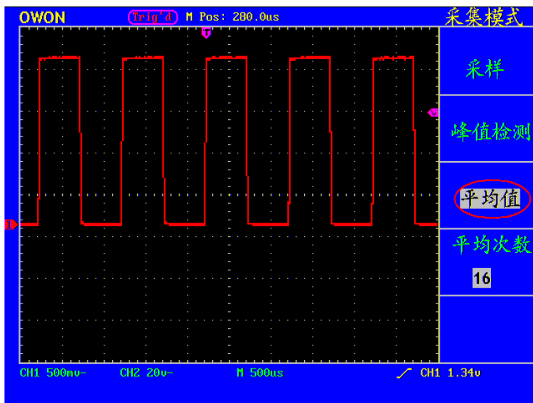
图 38: 平均次数为16次平均值方式, 去除噪声后的显示波形。
