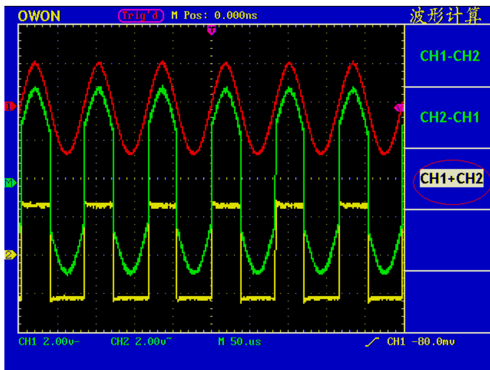
图 20 CH1+CH2 数学运算波形
