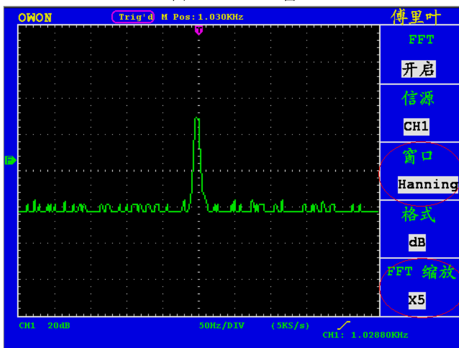
图22. Hanning窗
