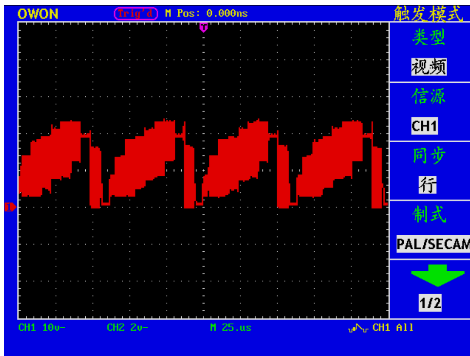
图 63 视频行触发波形
