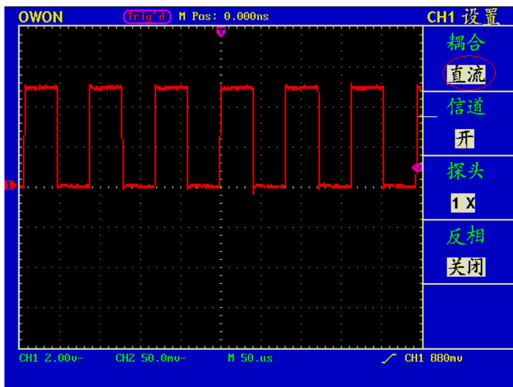
图 16 直流耦合波形图
