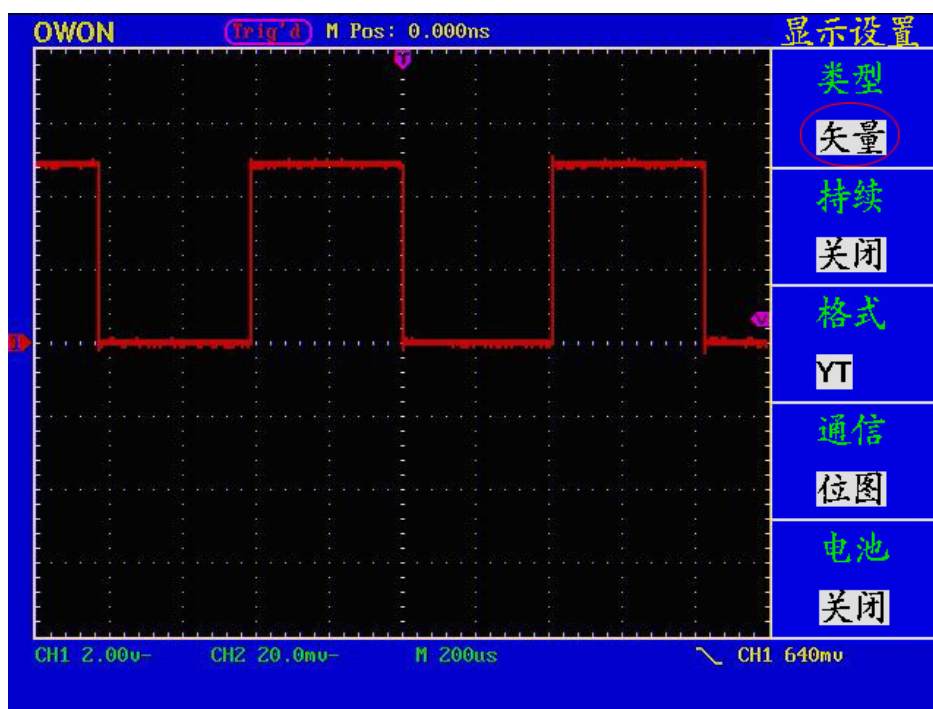
图 40： 矢量显示类型
