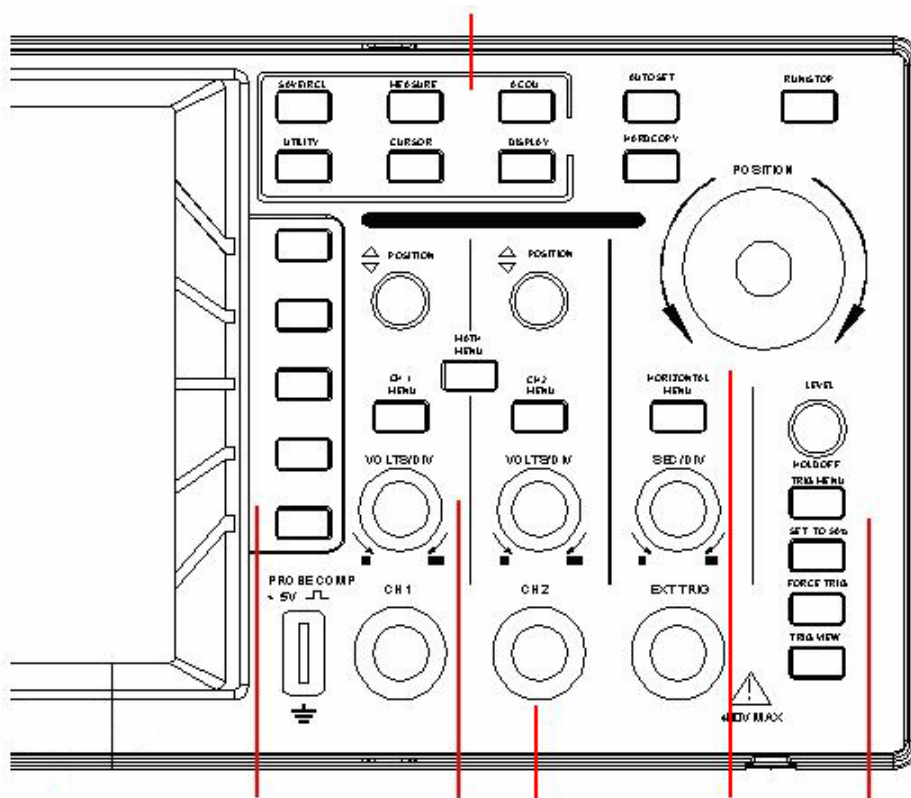
图 2 EDU 系列示波器面板操作说明图
