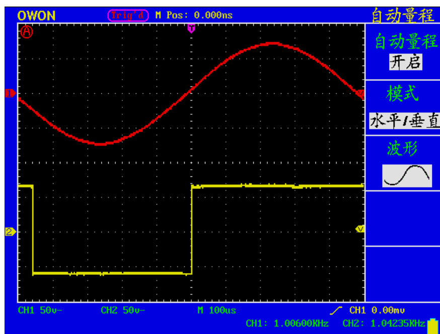
图 55 自动量程 水平/垂直模式单周期波形图
