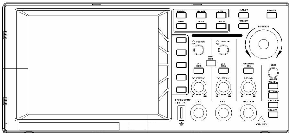
图 1 EDU 系列示波器前面板
