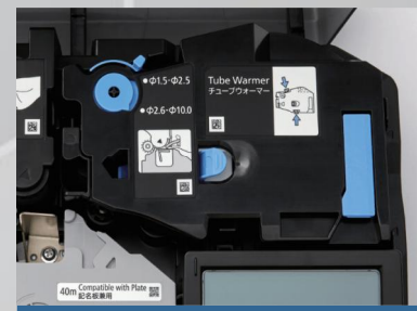
套管加热器(选配件)，支持在 5°C~15°C的低温环境中正常打印
