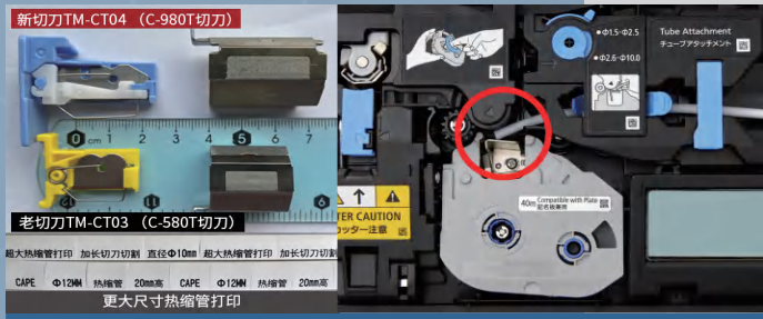
进料通道及切刀加大 支持大管打印—Φ1.5-Φ10 (0.5平方-25平方)
