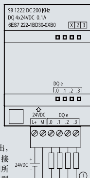
SB 1222 DC 200 kHz, 4 x 24 V DC 输出, 0.1 A
