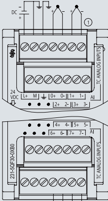
SM 1231 8 x 16 位热电偶模拟量输入
