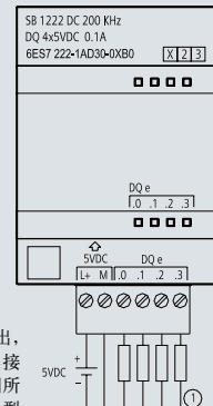
SB 1222 DC 200 kHz, 4 x 5 V DC 输出, 0.1 A
