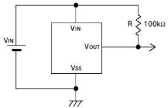
N-ch Open Drain 输出
