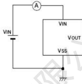
电路 4
