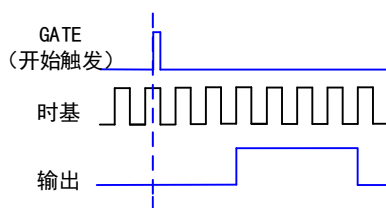
图 6-8-2 具有启动触发的单脉冲生成
