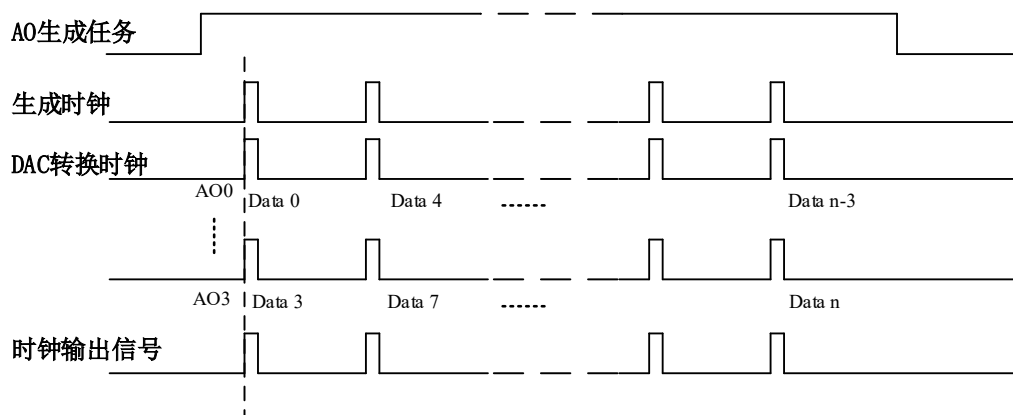
图 5-6-2 内时钟时序图
