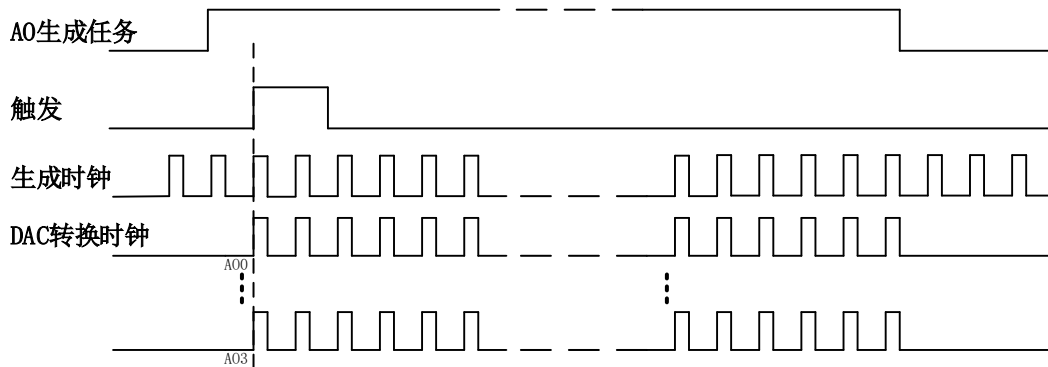
图5-7-3 内、外时钟连续采样
