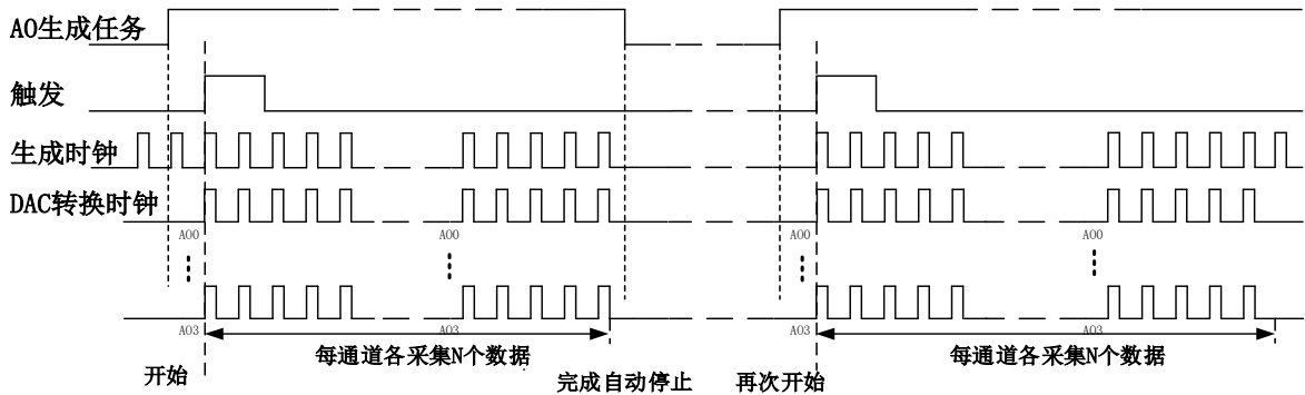
图5-7-2 内、外时钟有限点采样
