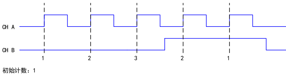
图 6-7-5 单脉冲编码
