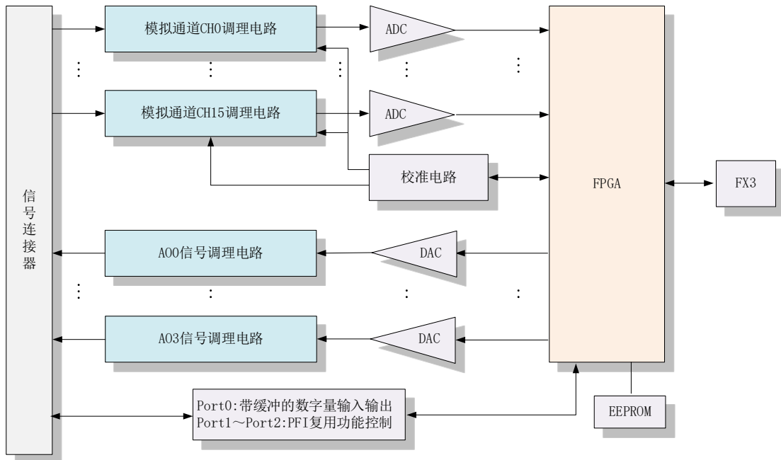
图2-2-1 USB2871_2(A/B/C)系统框图
