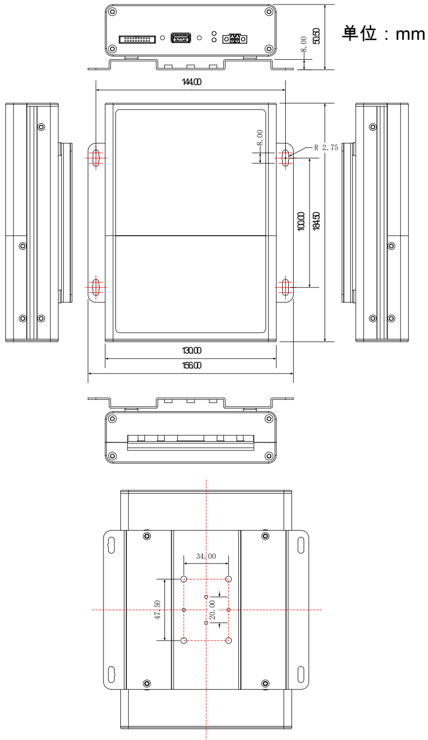
图 3-2-1 USB2871_2(A/B/C)-D 外壳尺寸图
