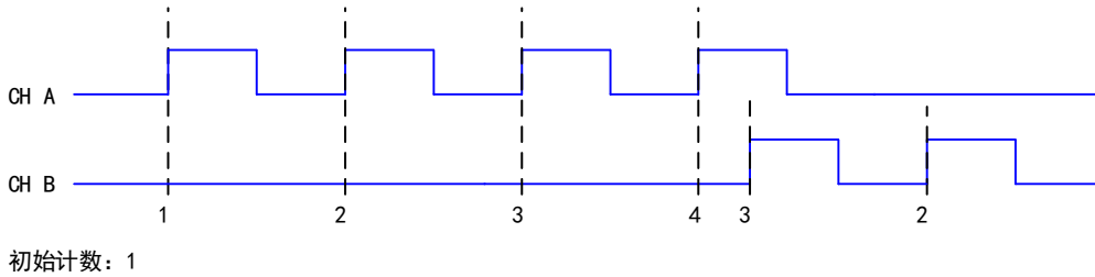
图 6-7-4 双脉冲编码
