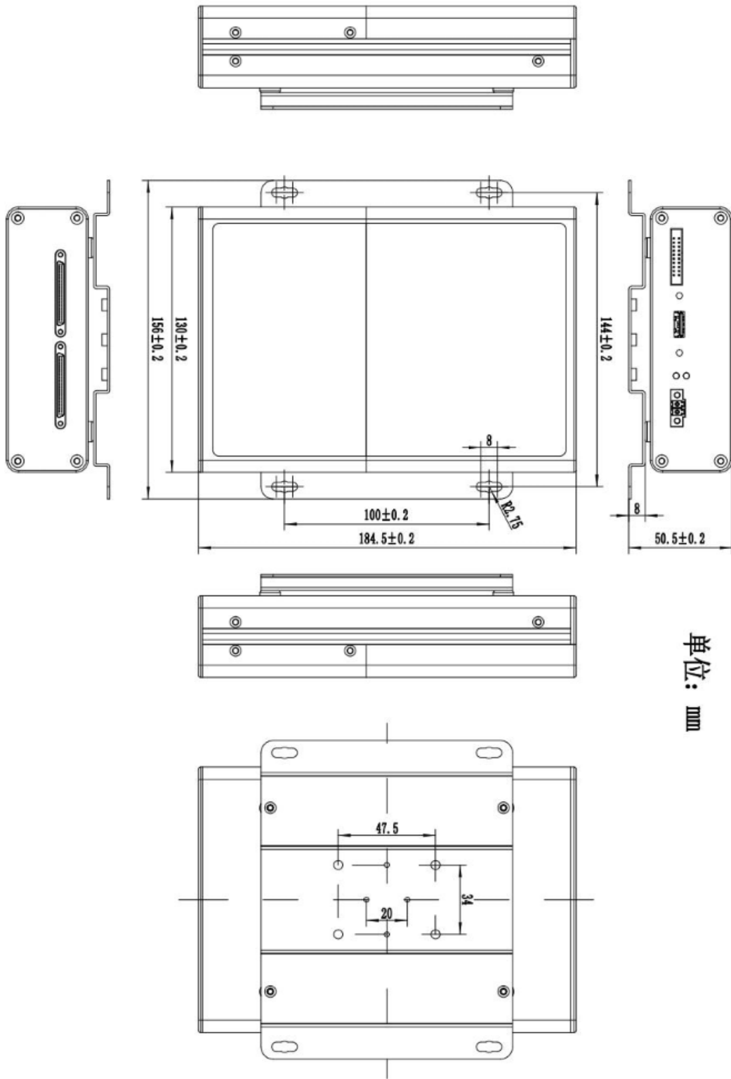
图 3-2-2 USB2871_2(A/B/C)-V 外壳尺寸图
