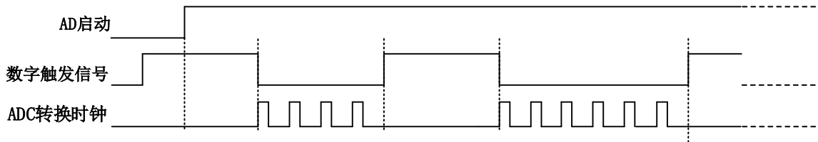
图 8-2-8 暂停触发—高电平暂停
