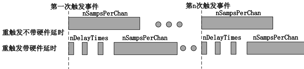
图 8-2-5 AI 重触发
