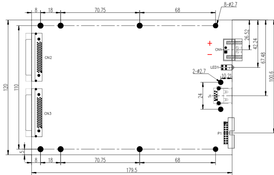
图 3-2-3 USB2871_2(A/B/C)板卡内部尺寸图
