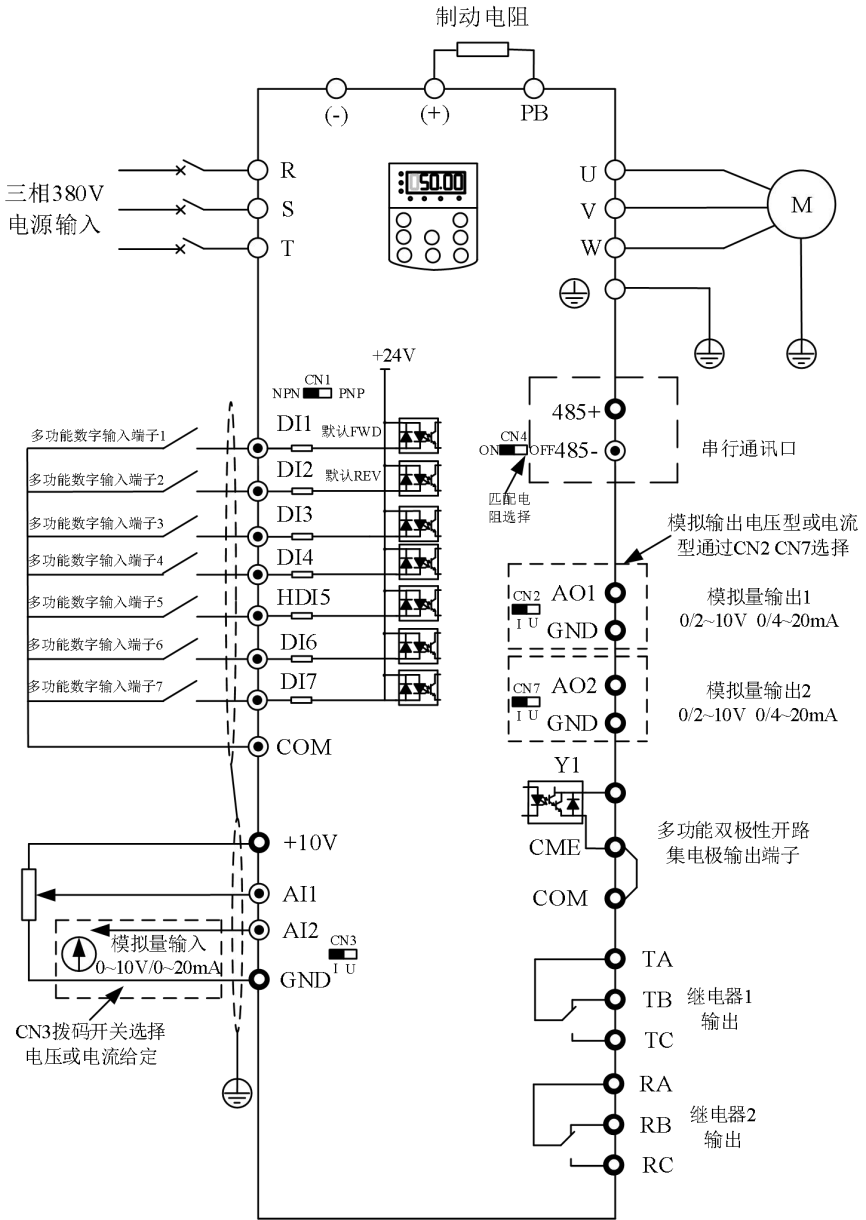
图 3-2. (4T/7T) 30kW 以下三相变频器
