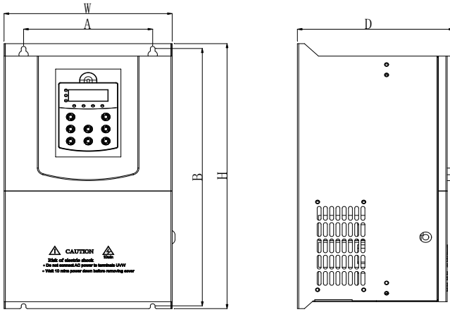
图 2-5. (4T) 18~37KW 钣金机箱外形尺寸及安装尺寸示意图 (7T) 11~15KW 钣金机箱外形尺寸及安装尺寸示意图
