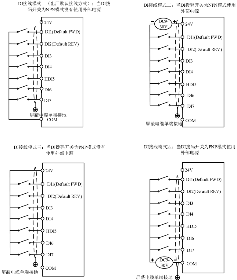
图3-7. 四种不同模式下数字输入端子接线图
