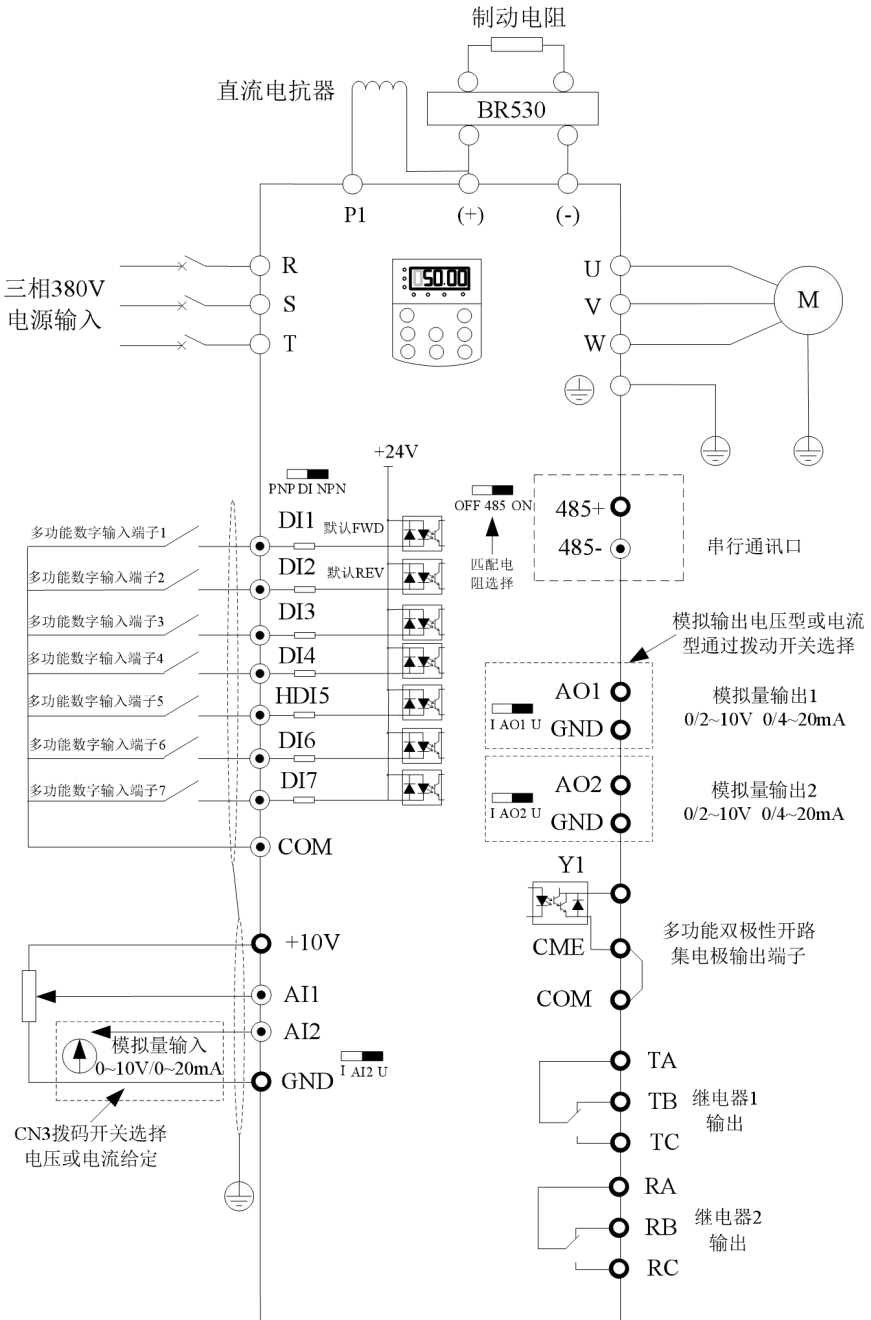
图 3-4. (4T) 75Kw 及以上三相变频器
