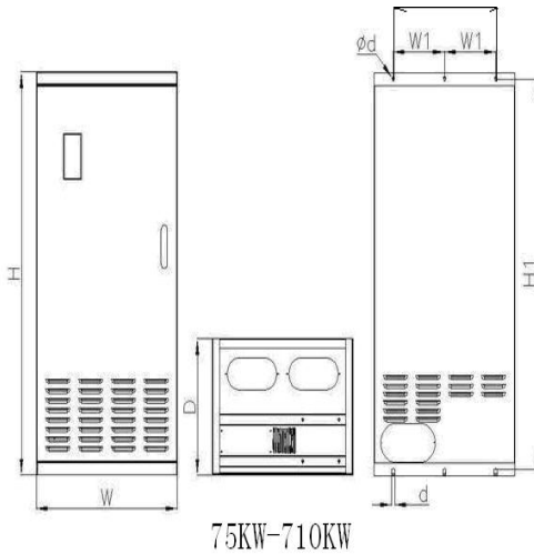
图 2-8. (7T) 75KW 以上变频器外型尺寸及安装尺寸示意图
