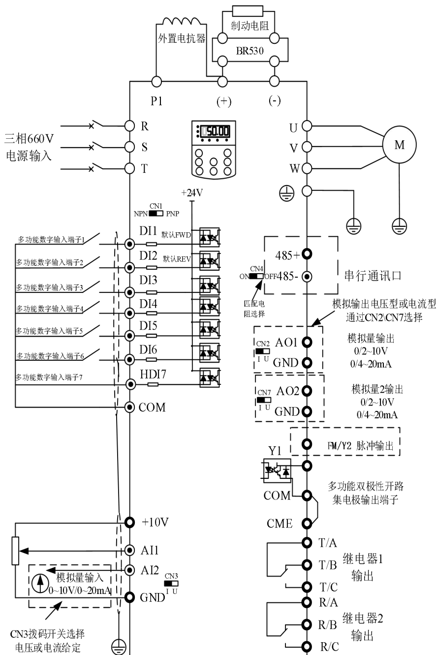
图 3-5. (7T)75Kw 及以上三相变频器
