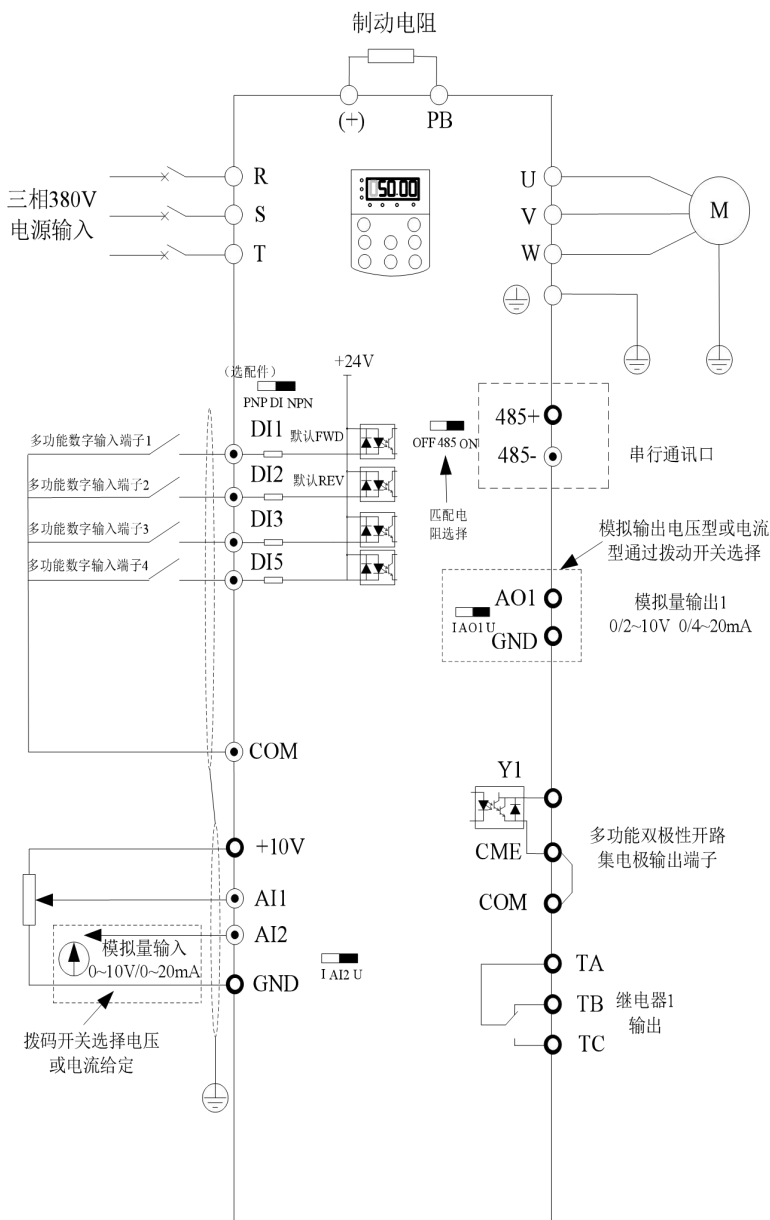
图 3-1. 1.5kW 以下三相变频器
