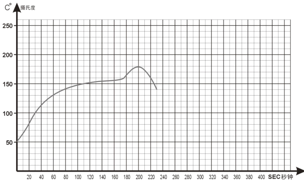
参考回流曲线：无铅低温锡膏 Sn42Bi58
