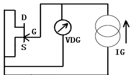
5.6.1.3 IDOFF (漏极的关断电流)
