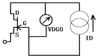
5.6.1.2 BVGSS (漏源极短路情况下, 源极-栅极的击穿电压)
