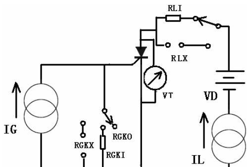
5.4.1.10 IL (擎住电流)
