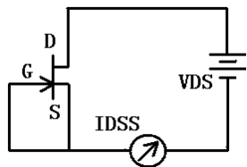
5.6.1.6 IGSS (漏极-源极短路情况下, 栅极-源极的漏电流)
