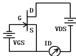
5.6.1.4 IDG0 (源极开路情况下, 漏极-栅极的漏电流)
