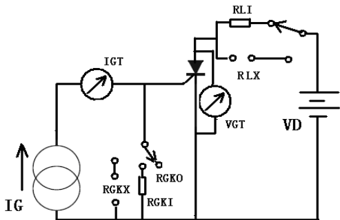
5.4.1.8 IGT (在特别条件下, 门极触发电流)
