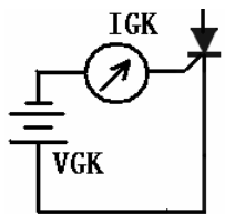
5.4.1.7 VGT (在特别条件下, 门极触发电压)
