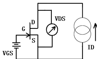
5.6.1.7 VDSON (漏极-源极开启电压)
