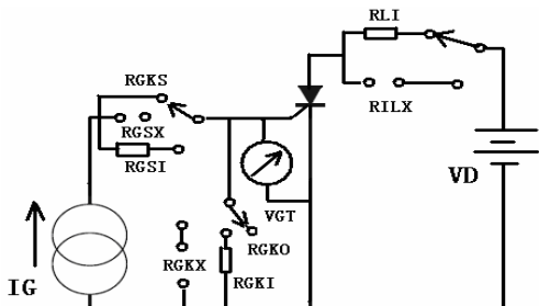
5.4.1.8 IGT (在特别条件下, 门极触发电流)
